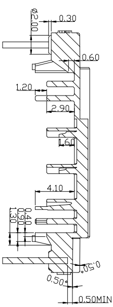
C-C(2:1)
